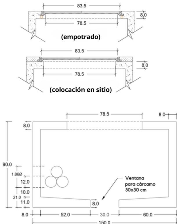
Corte A-A
