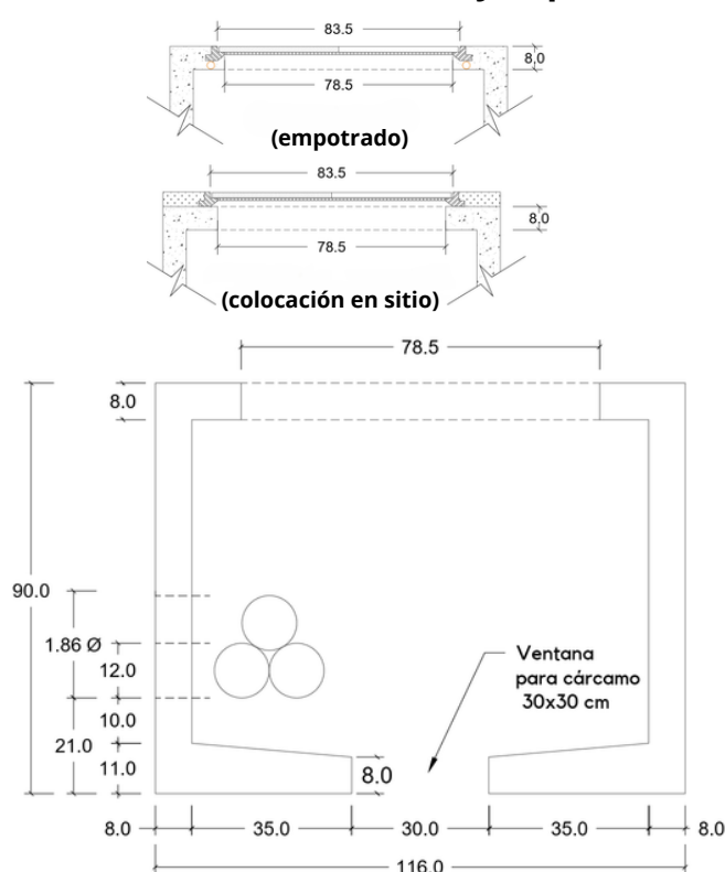
Corte A-A
