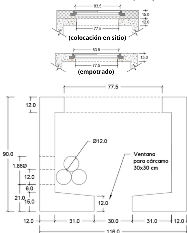
Corte A-A
